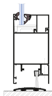
Prahová lišta s kartáčem
