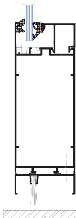
Bezprahové dveře s kartáčem
