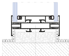
Montáž u podhledu
