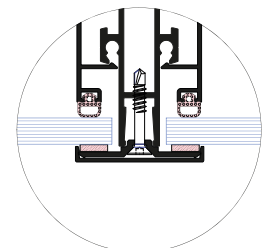
Listwa przykrycana
