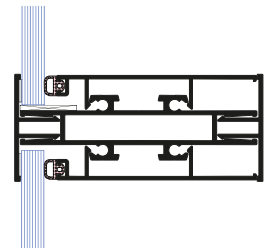
Jednoduché zasklení
