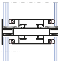
dvojsklo
