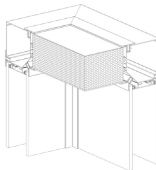
Možnost realizace boxů včetně střeš
