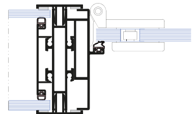
Celoskleněné dveře
