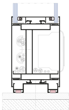
Montáž na podlaze s profilem pro el. rozvody
