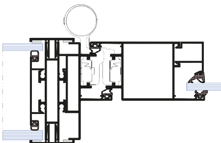
Hliníkové dveře ACS 50
